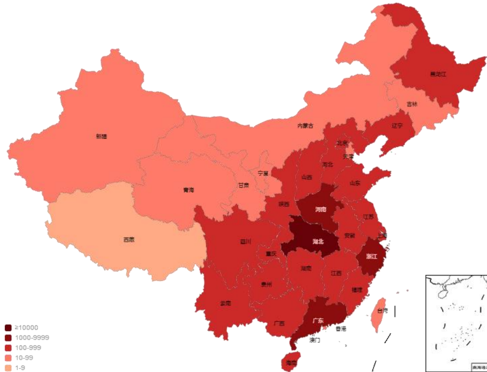
图2 本次 NCP 爆发的地区图
